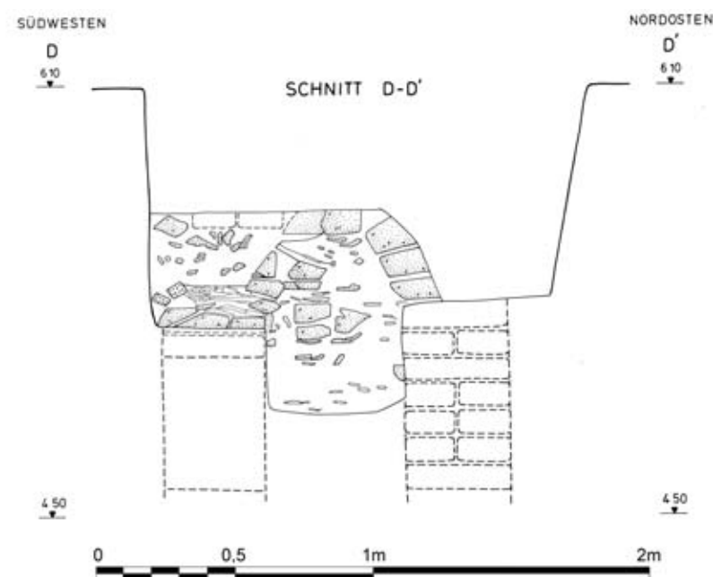
Abb. 392 F/I-o/20-Grab 11, Schnitt D-D'
