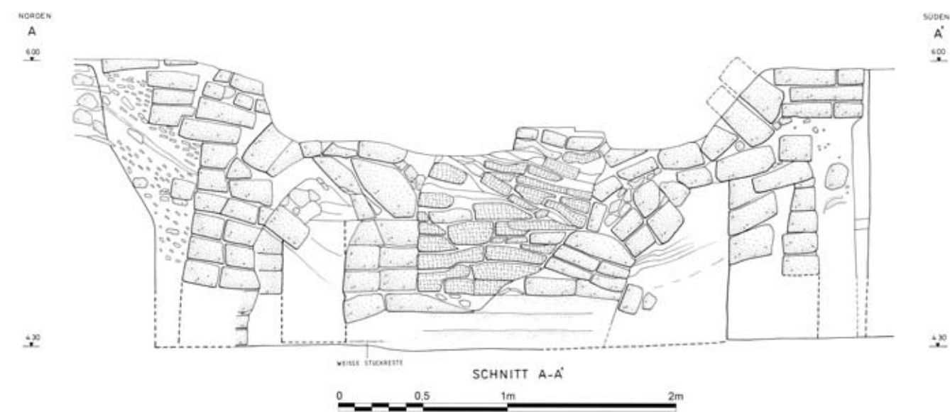
Abb. 344 F/I-m/18-Grab 2, Schnitt A-A'
