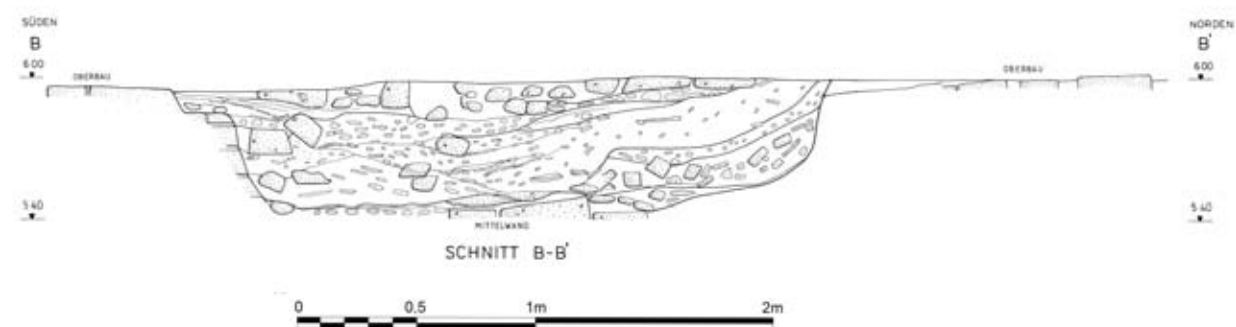
Abb. 345 F/I-m/18-Grab 2, Schnitt B-B'
