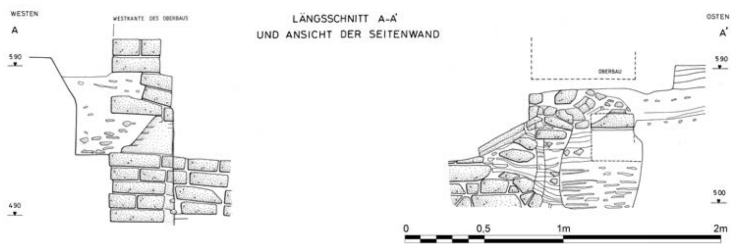
Abb. 388 F/I-o/20-Grab 11, Längsschnitt A-A'
