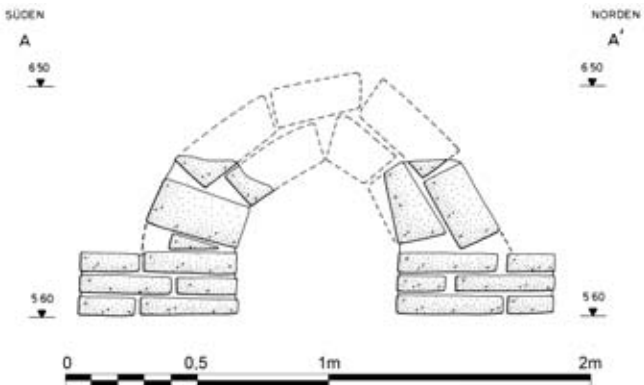
Abb. 351 F/I-n/17-Grab 3, Schnitt A–A’
