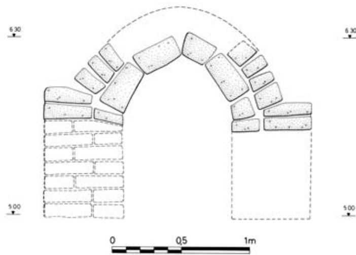
Abb. 361 F/I-o/17-Grav 1, Schnitt A–A' rekonstruiert
