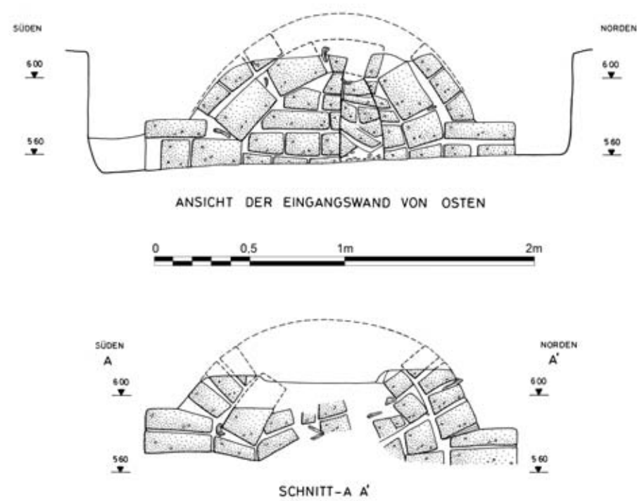
Abb. 360 F/I-o/17-Grav 1, Ansicht der Eingangswand von Osten und Schnitt A–A'
